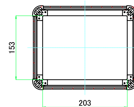
C-C ( 1 : 5.5 )
